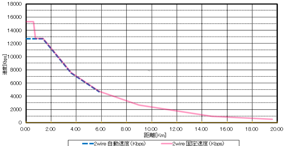
N51 距離と速度グラフ 線径0.9mm
